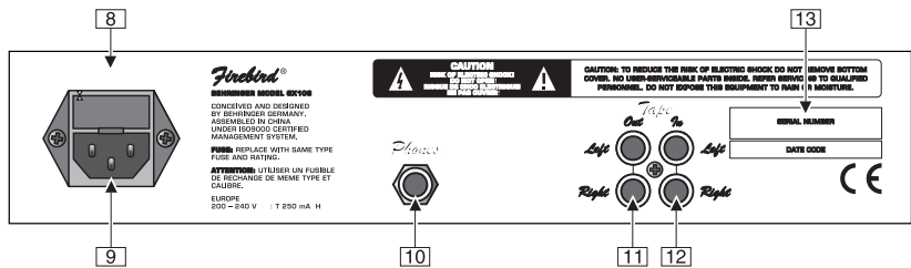
Fig. 1.2: Conexiones en el reverso
