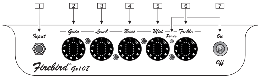
Fig. 1.1: Elementos de mando en la cara frontal
