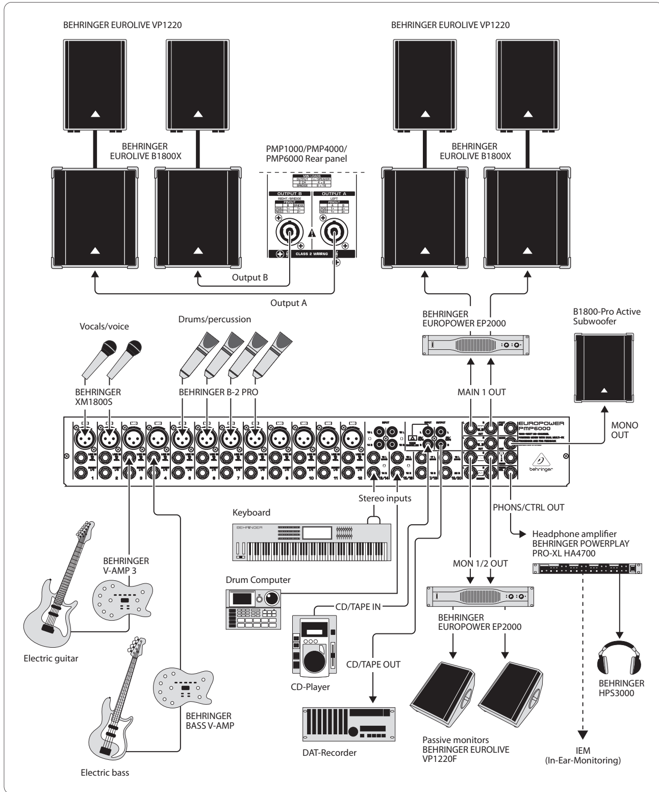
Fig. 5.5: Configuración ampliada
