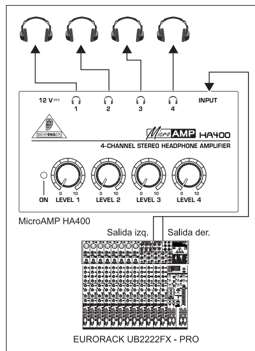
Cableado del HA400
