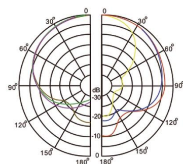
1kHz ■ 16kHz ■ 2kHz ■ CONDENSER/CONDENSADOR
