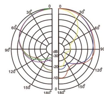
1kHz 2kHz 16kHz CONDENSER/CONDENSADOR
