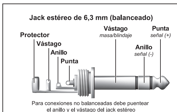
Fig. 5.2: Jack estéreo de 6,3 mm
