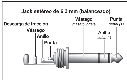
Fig. 5.4: Jack estéreo de 6,3 mm
