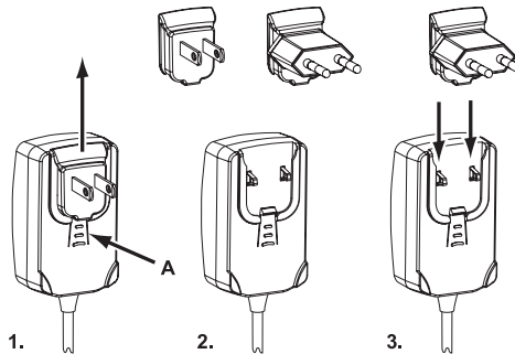
Fig. 1.1: Cambio de clavija del adaptador de corriente
