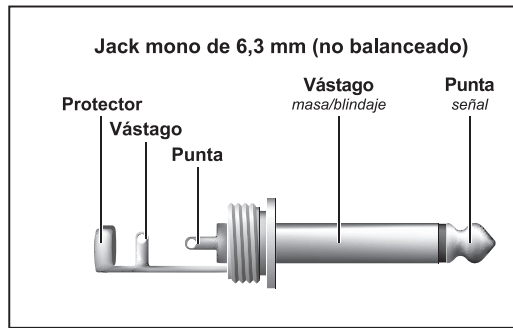
Fig. 5.3: Jack mono de 6,3 mm
