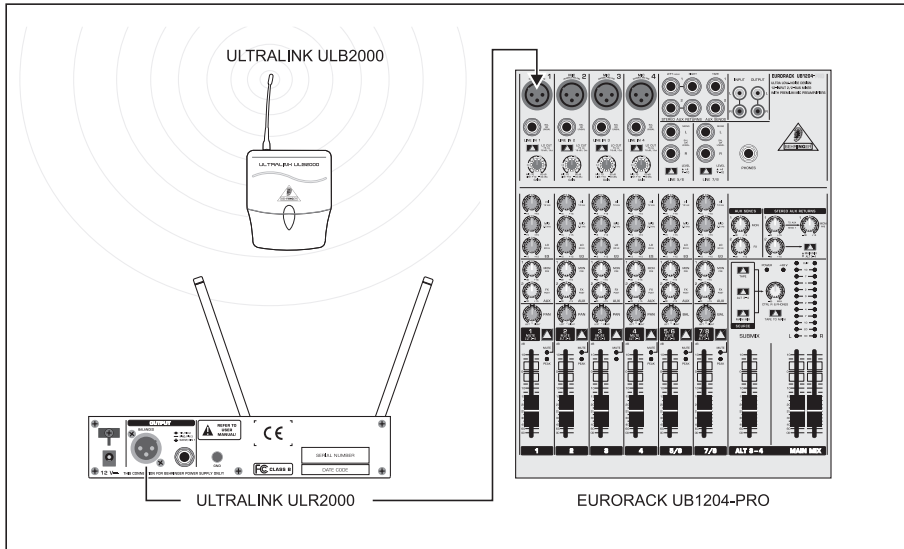
Fig. 4.1: Conexión del receptor ULR2000 y del micrófono ULB2000
