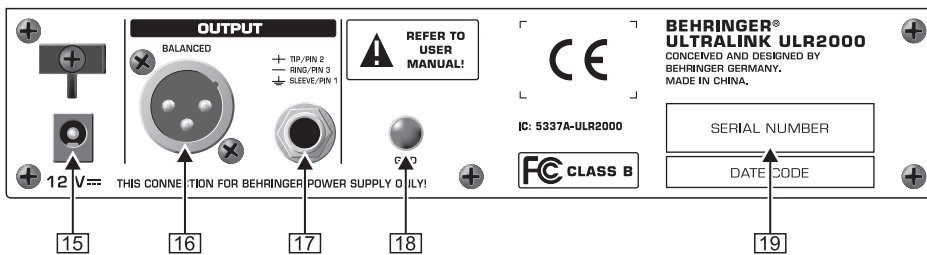
Fig. 2.3: Parte posterior del ULR2000
