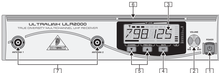
Fig. 2.1: Parte delantera del ULR2000
