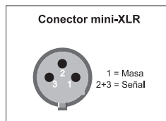
Fig.5.5: Conector mini XLR del ULB2000
