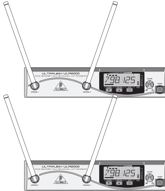
Fig. 5.1: Colocación de dos ULR2000 a manera de pila
